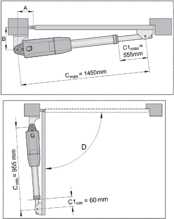
twist 350 A/B 尺寸表
