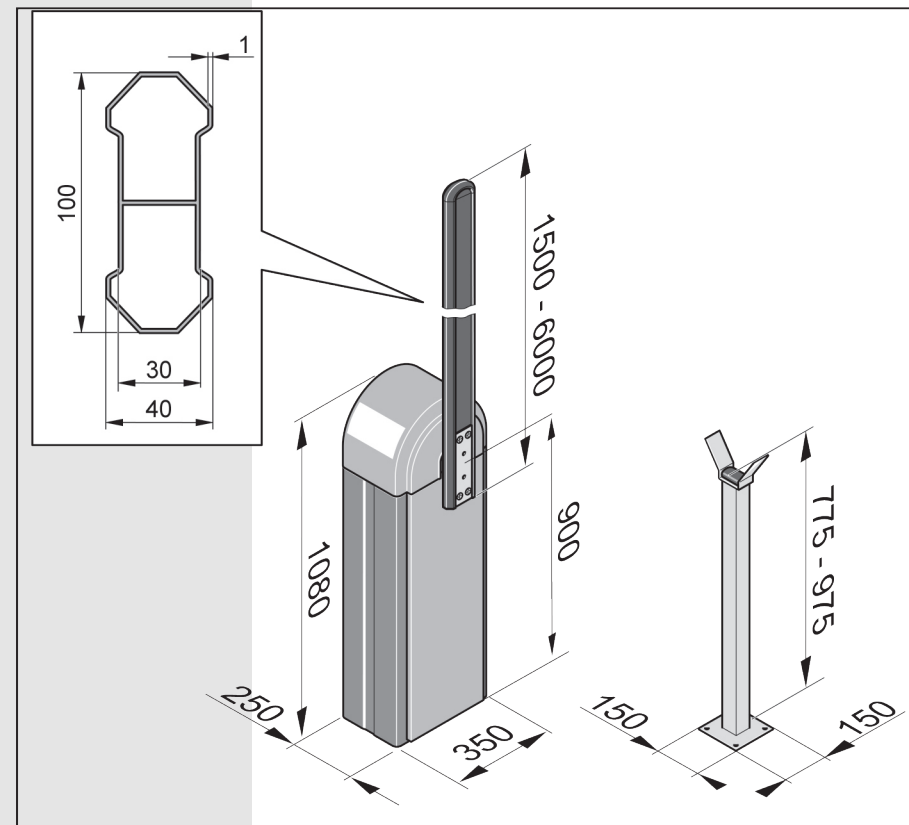
尺寸图
