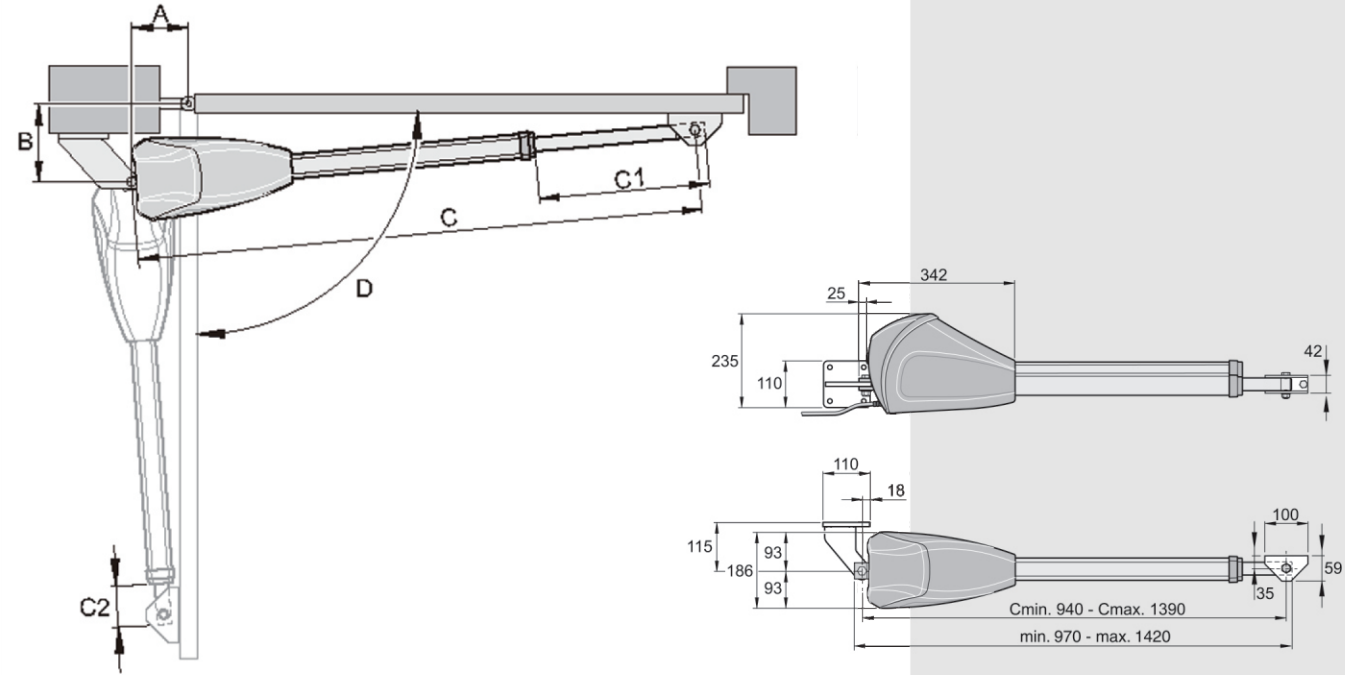
twist XL 尺寸图
