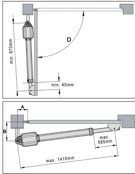
twist 200 EL A/B 尺寸表
