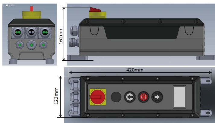
控制盒尺寸
