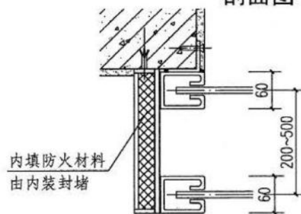
剖面图
