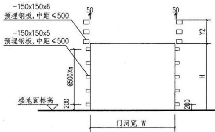
钢筋混凝土门框预埋件示意图
