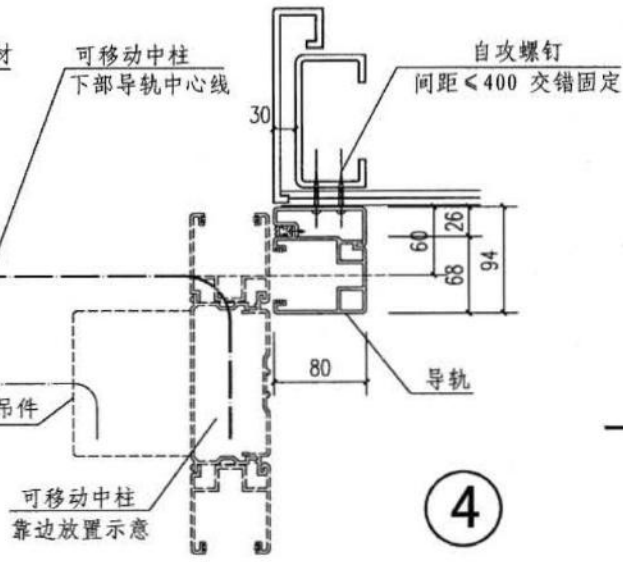
透明分节门安装节点示意图
