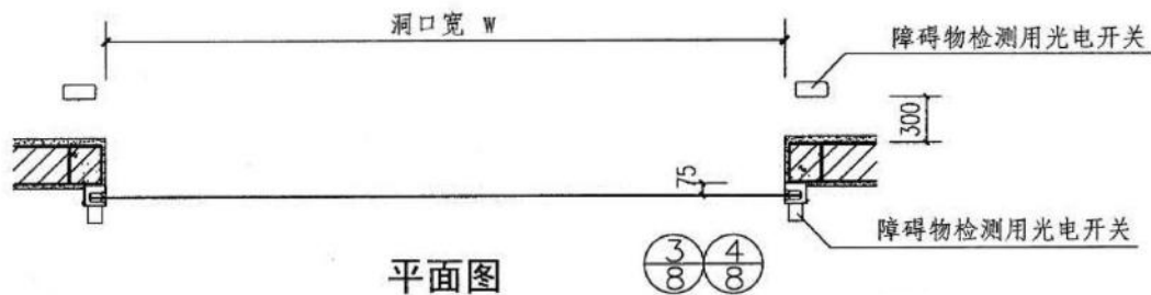
快速软帘卷门安装示意图
