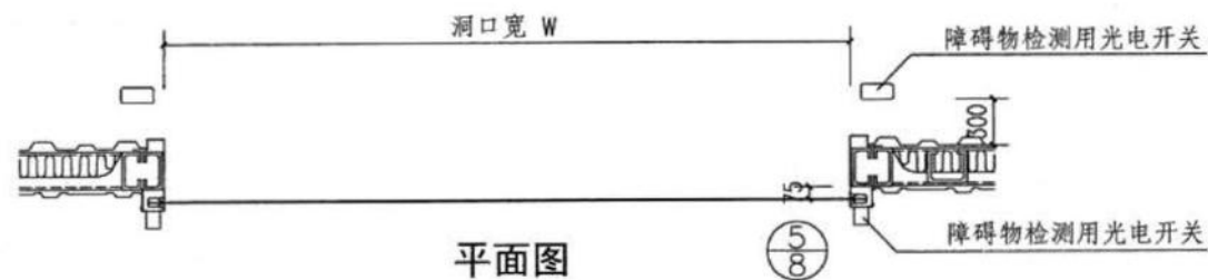
快速软帘卷门安装示意图
