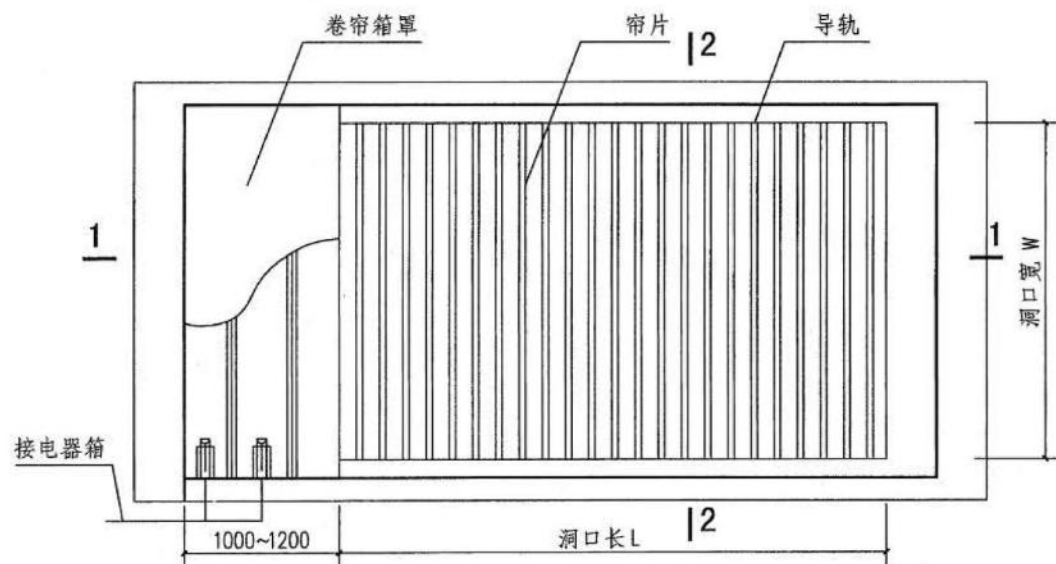
平面图
