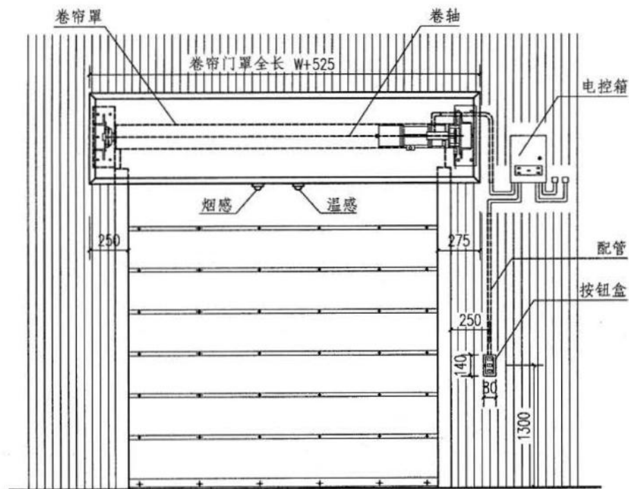
内立面图
