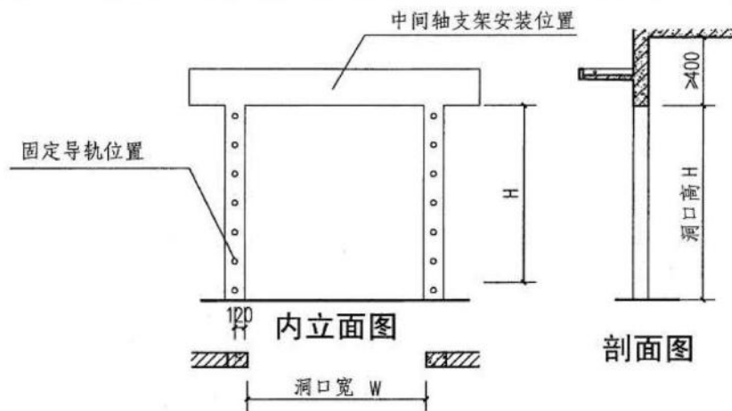
低扬程型混凝土门框平面图
