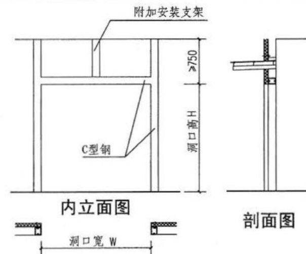
标准型钢结构门框平面图
