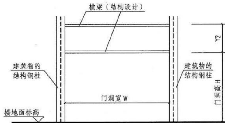
钢结构门框示意图 (二)
