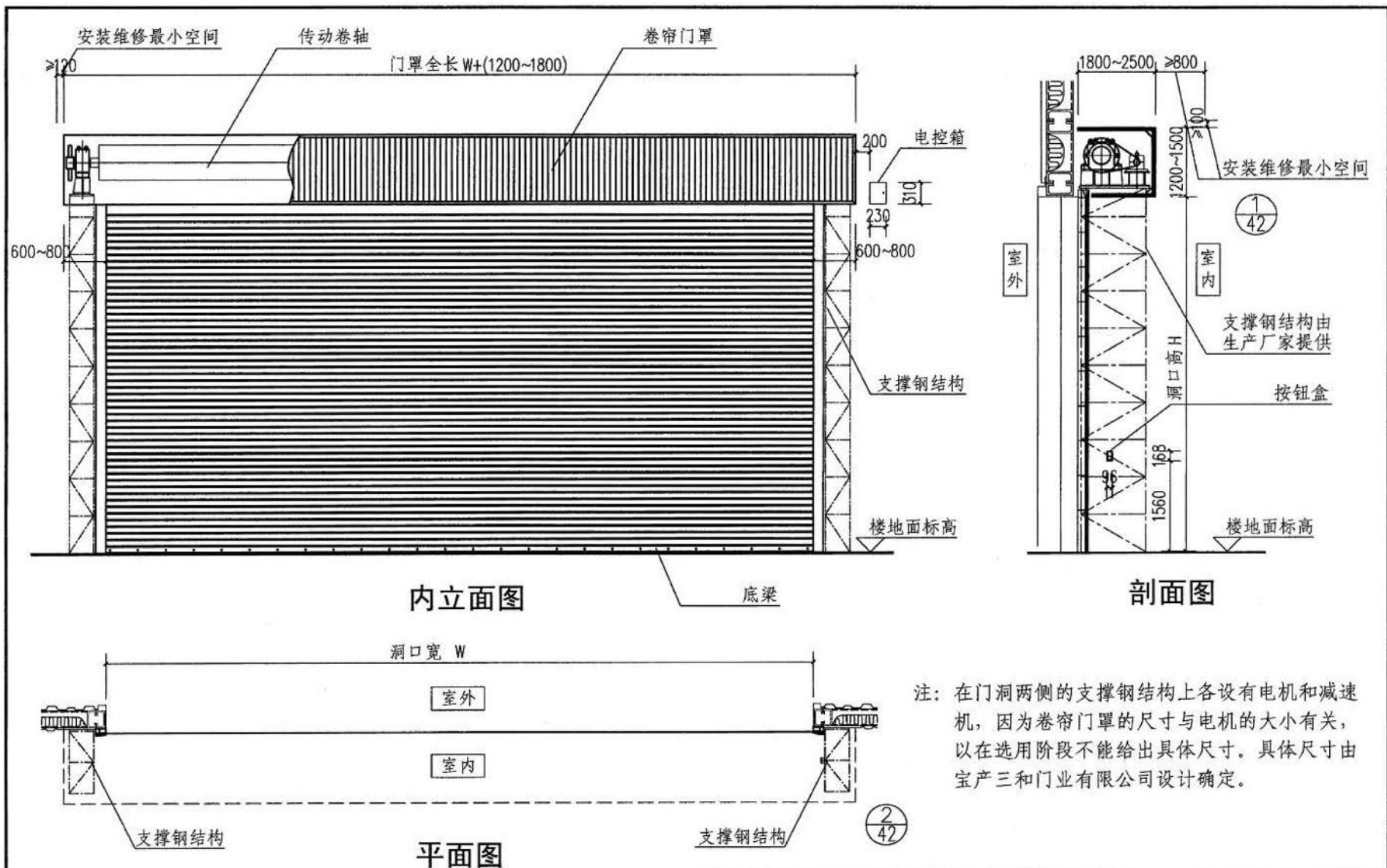
超重型卷帘门安装示意图
