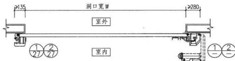
平面图
