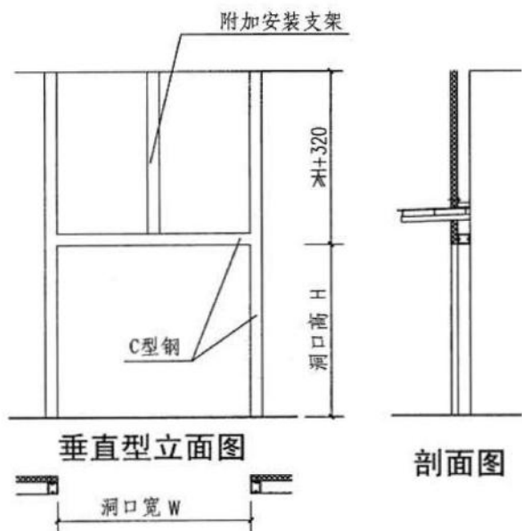
垂直型钢结构门框平面图
