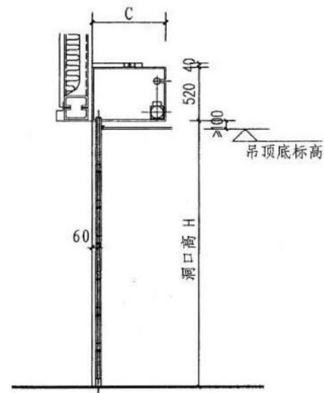
剖面图
