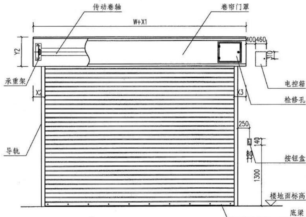
内立面图
