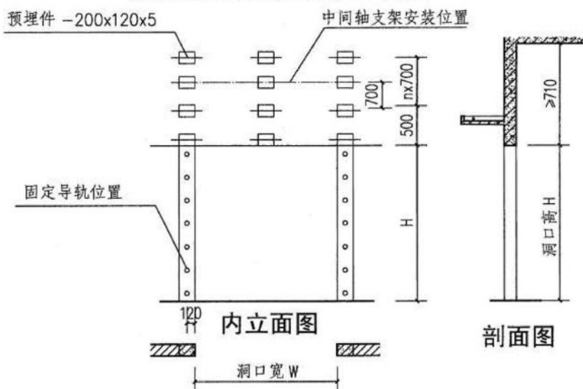
高扬程型混凝土门框平面图
