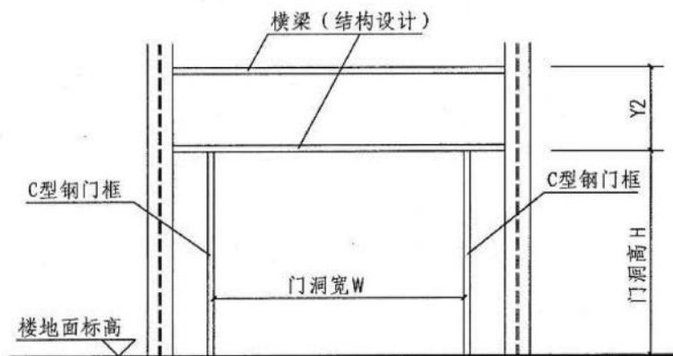
钢结构门框示意图 (一)
