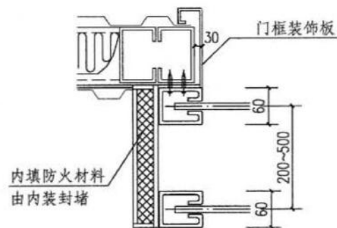
双轨无机布防火卷帘门安装示意图
