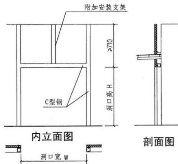
高扬程型钢结构门框平面图
