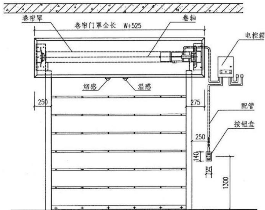
内立面图
