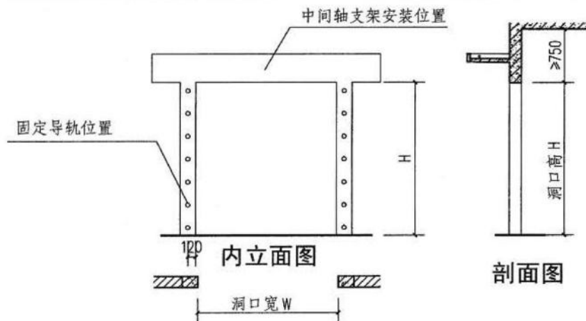
标准型混凝土门框平面图
