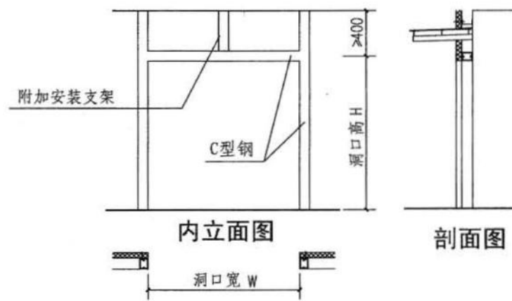
低扬程型钢结构门框平面图
