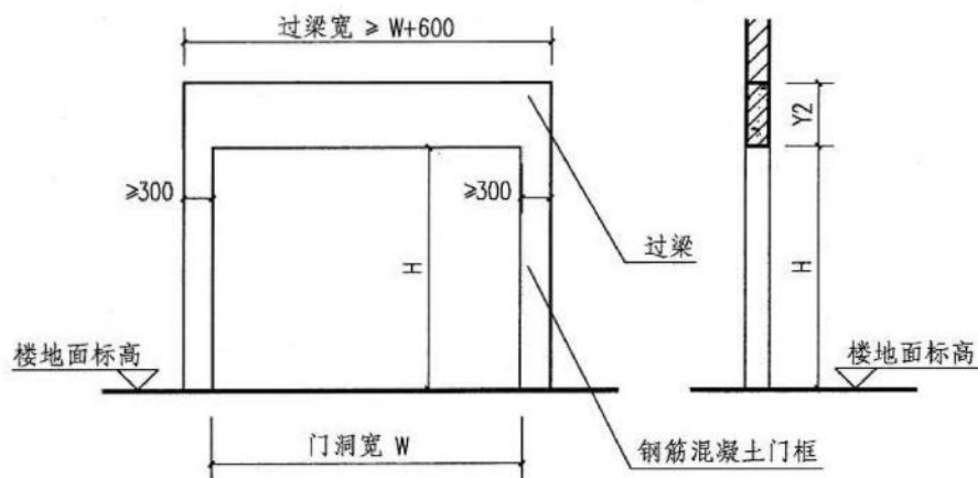
钢筋混凝土门框示意图
