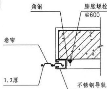
剖面图
