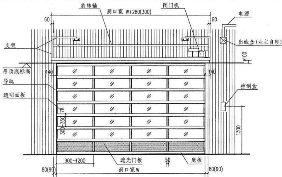
内立面图
