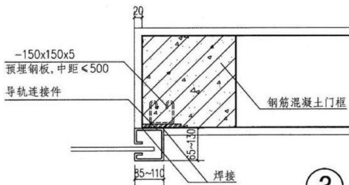
钢筋混凝土门框节点图
