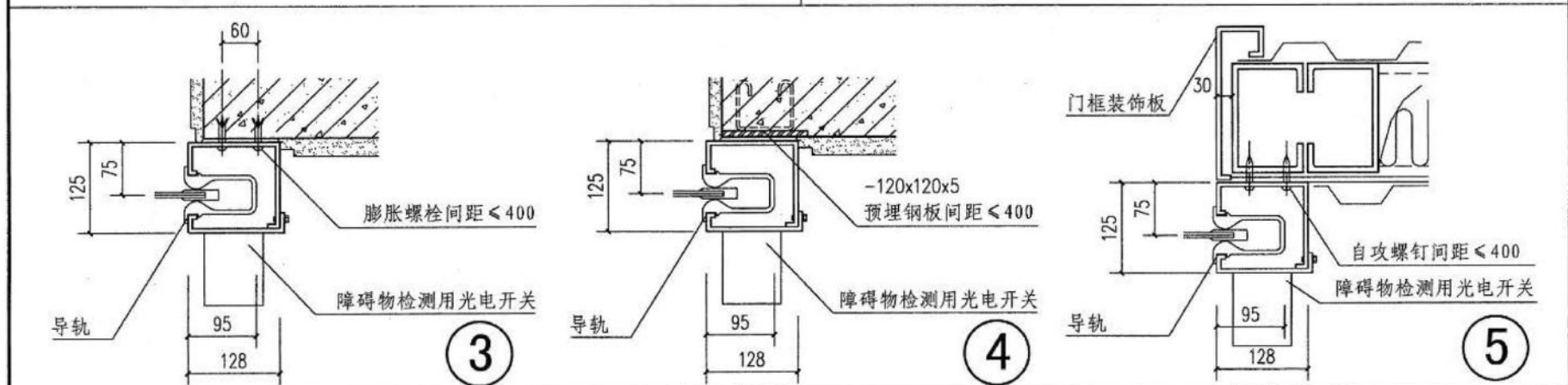
快速软帘卷门安装节点示意图
