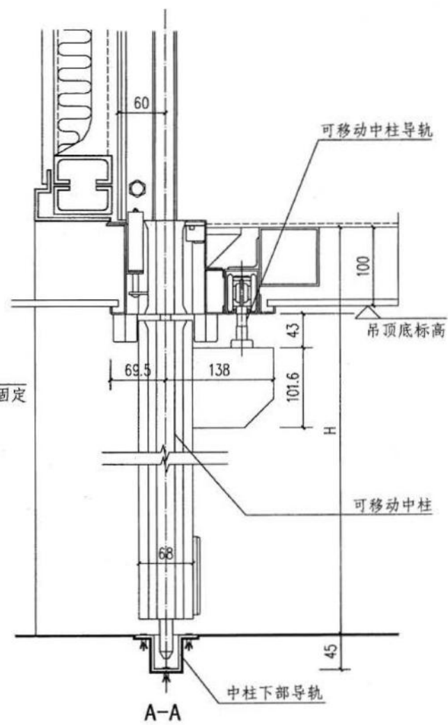
透明分节门安装节点示意图
