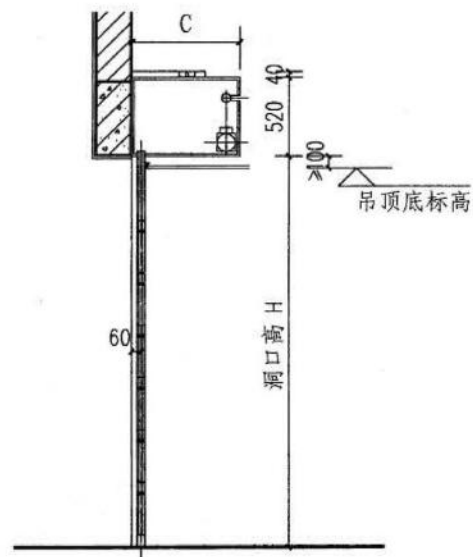
剖面图
