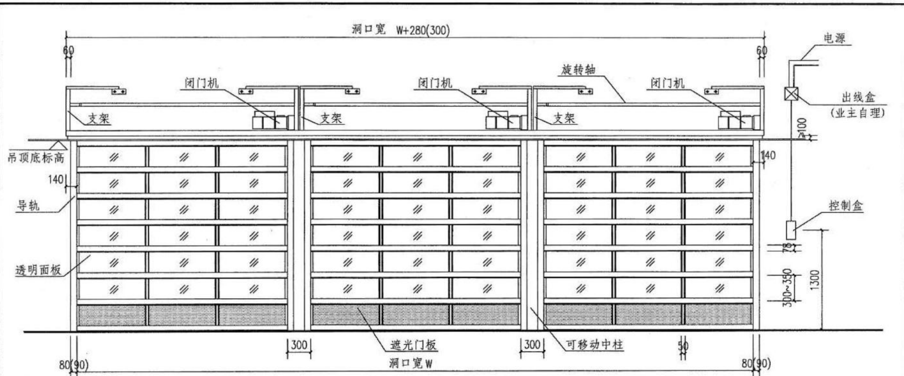
内立面图
