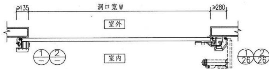
平面图
