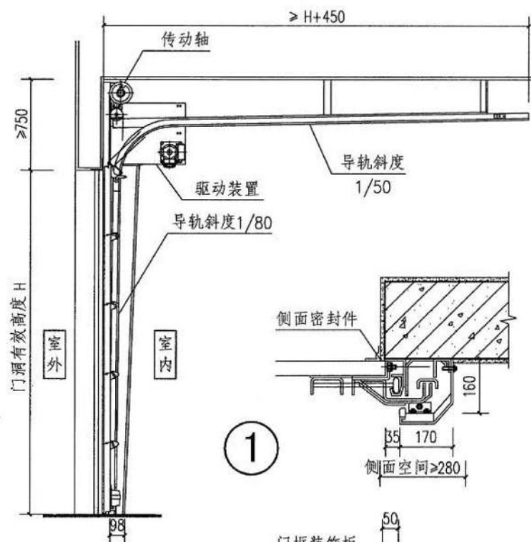
剖面图
