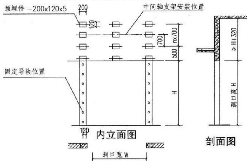
垂直型混凝土门框平面图
