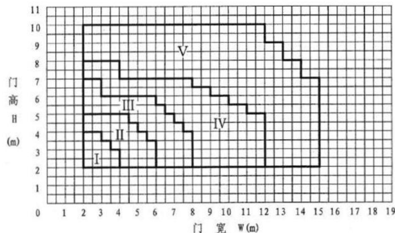
复合帘片卷帘门规格编号
