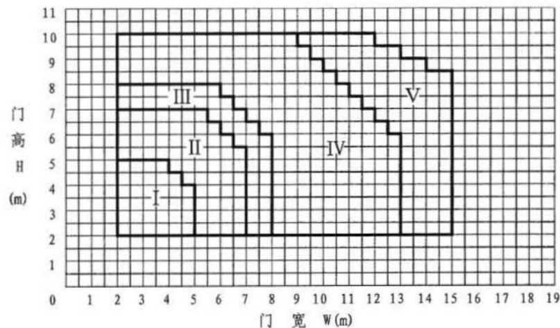
单片帘片卷帘门规格编号
