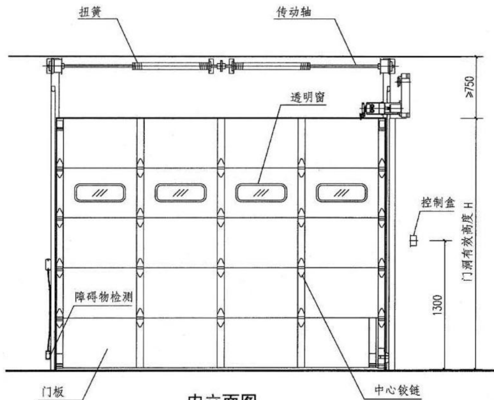
内立面图
