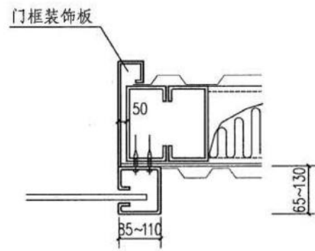
钢结构门框节点图
