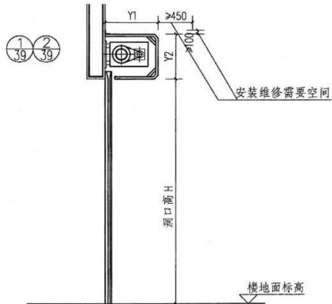
剖面图
