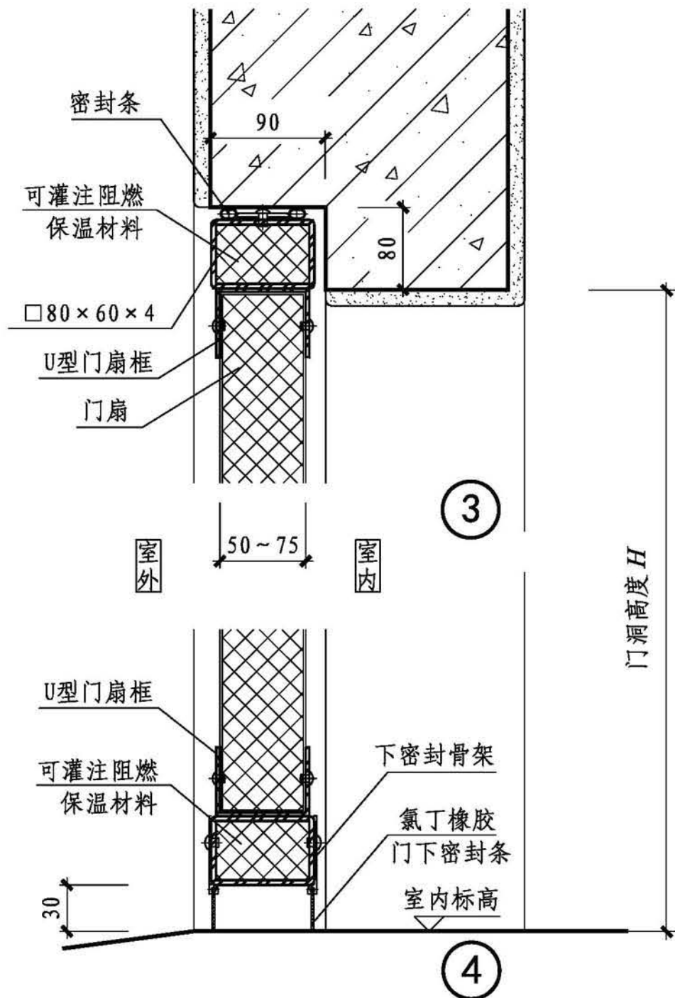
平开门（无门框）详图
