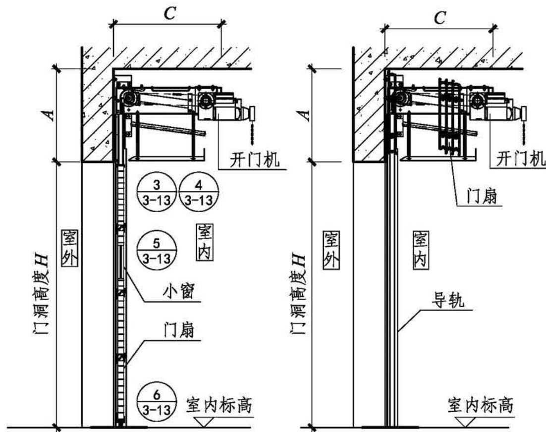
1-1剖面图 (门关闭状态)
