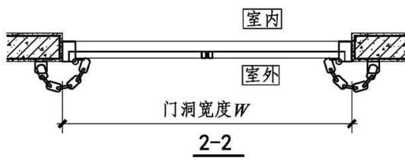
平开门防脱链做法示意图
