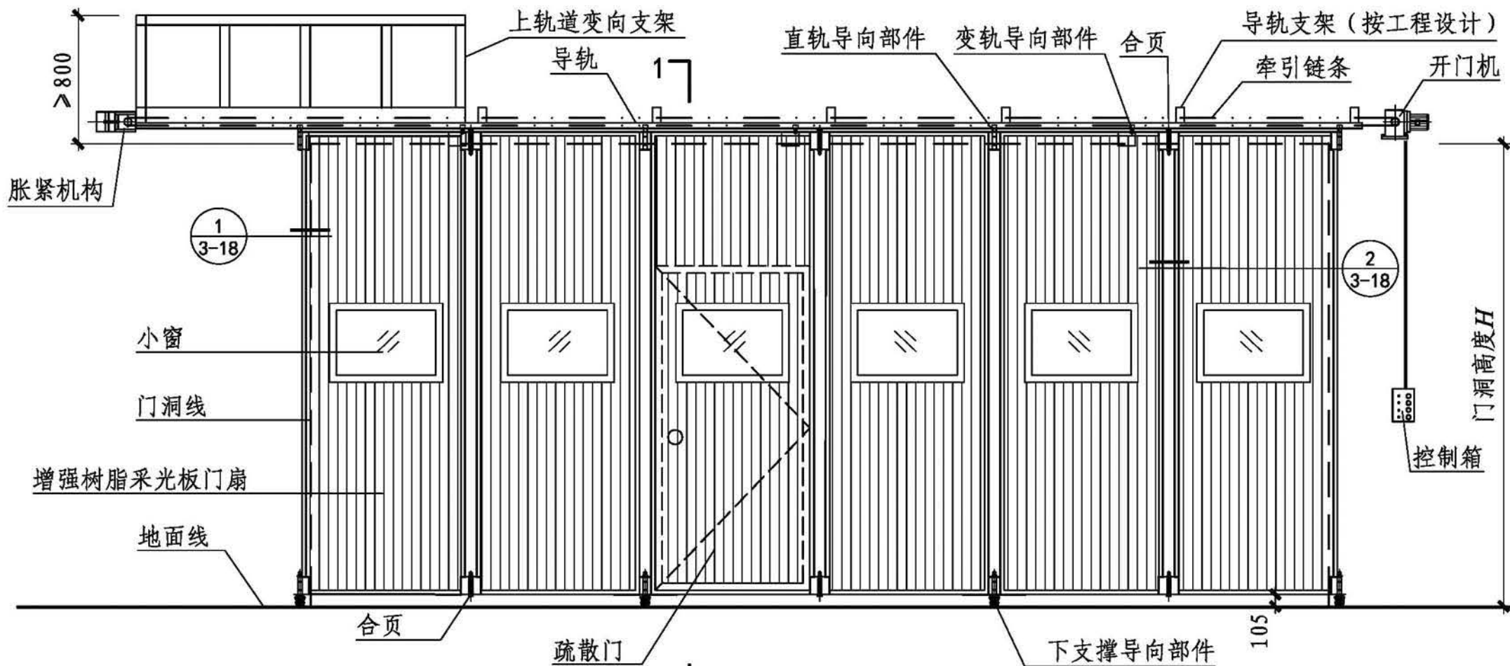
内立面图
