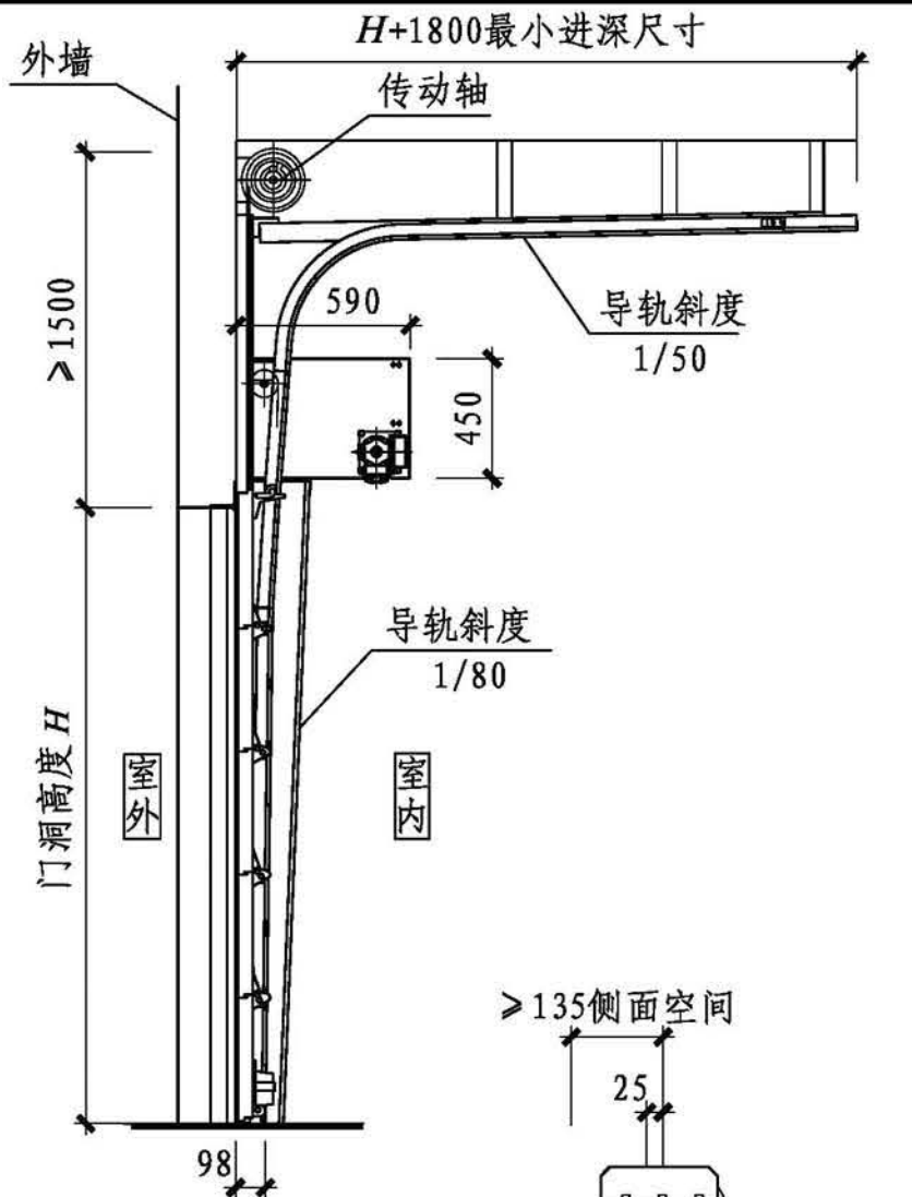
1-1剖面图
