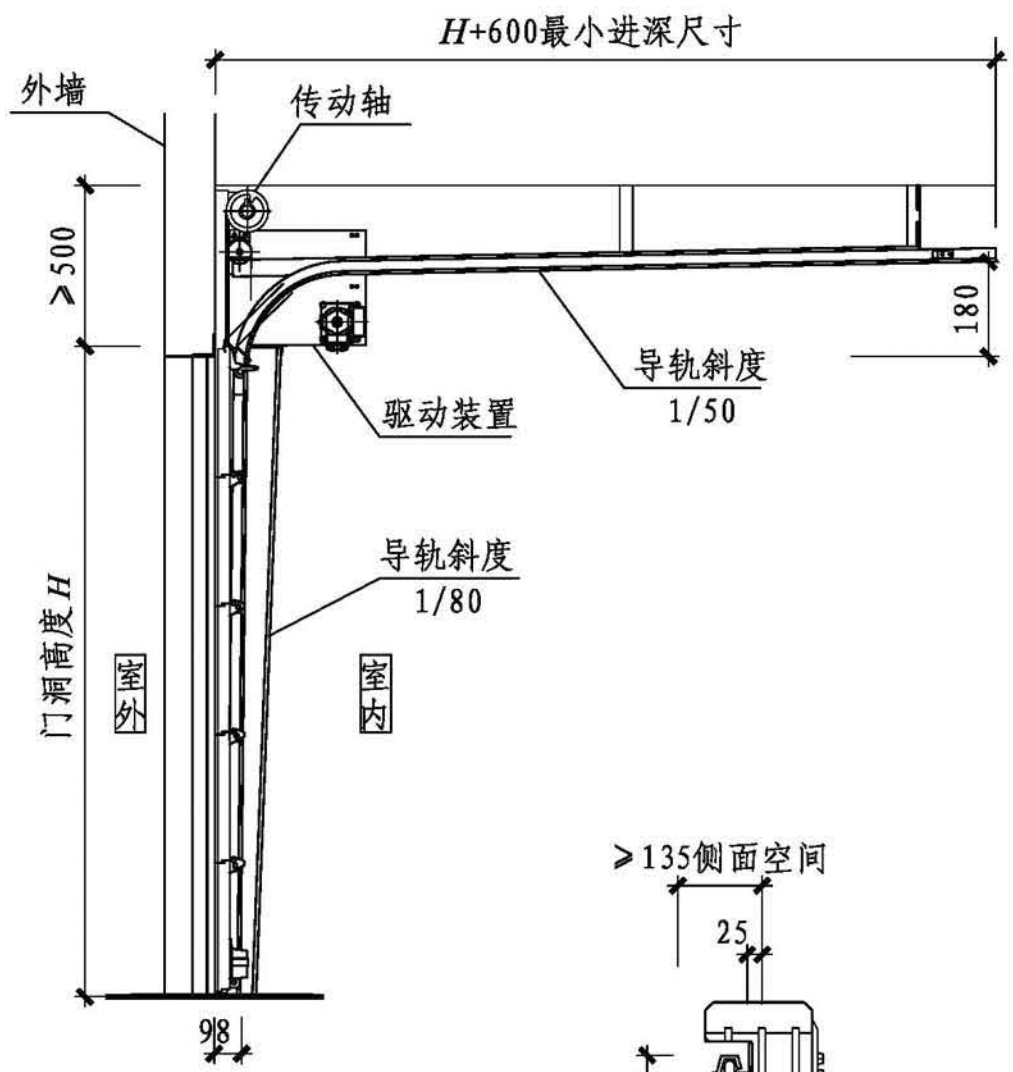
1-1剖面图
