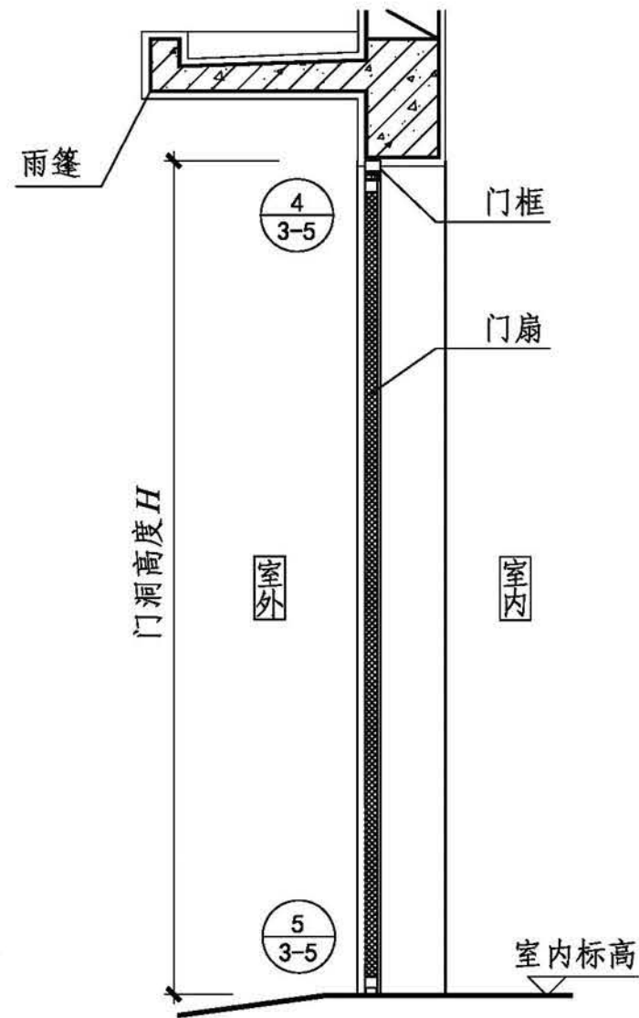
1-1剖面图
