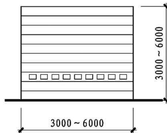
增强树脂板上叠门
