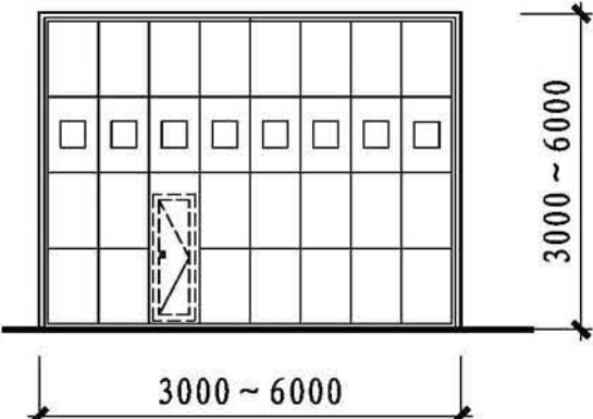
滑升门 (带小门)
