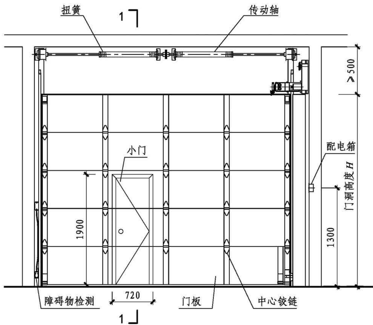
内立面图
