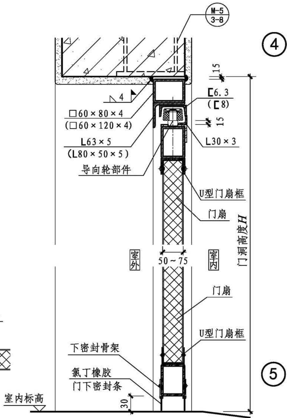
折叠门（手动）详图
