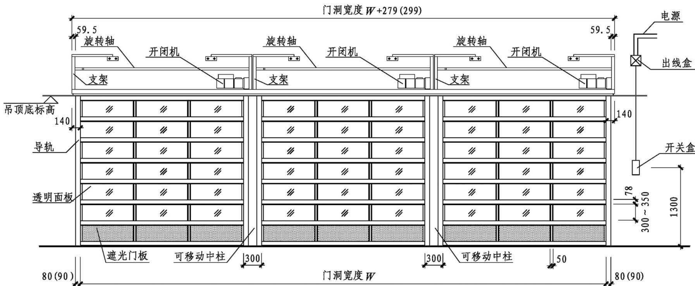
内立面图
