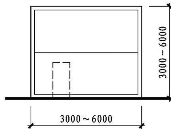
上折门立面
