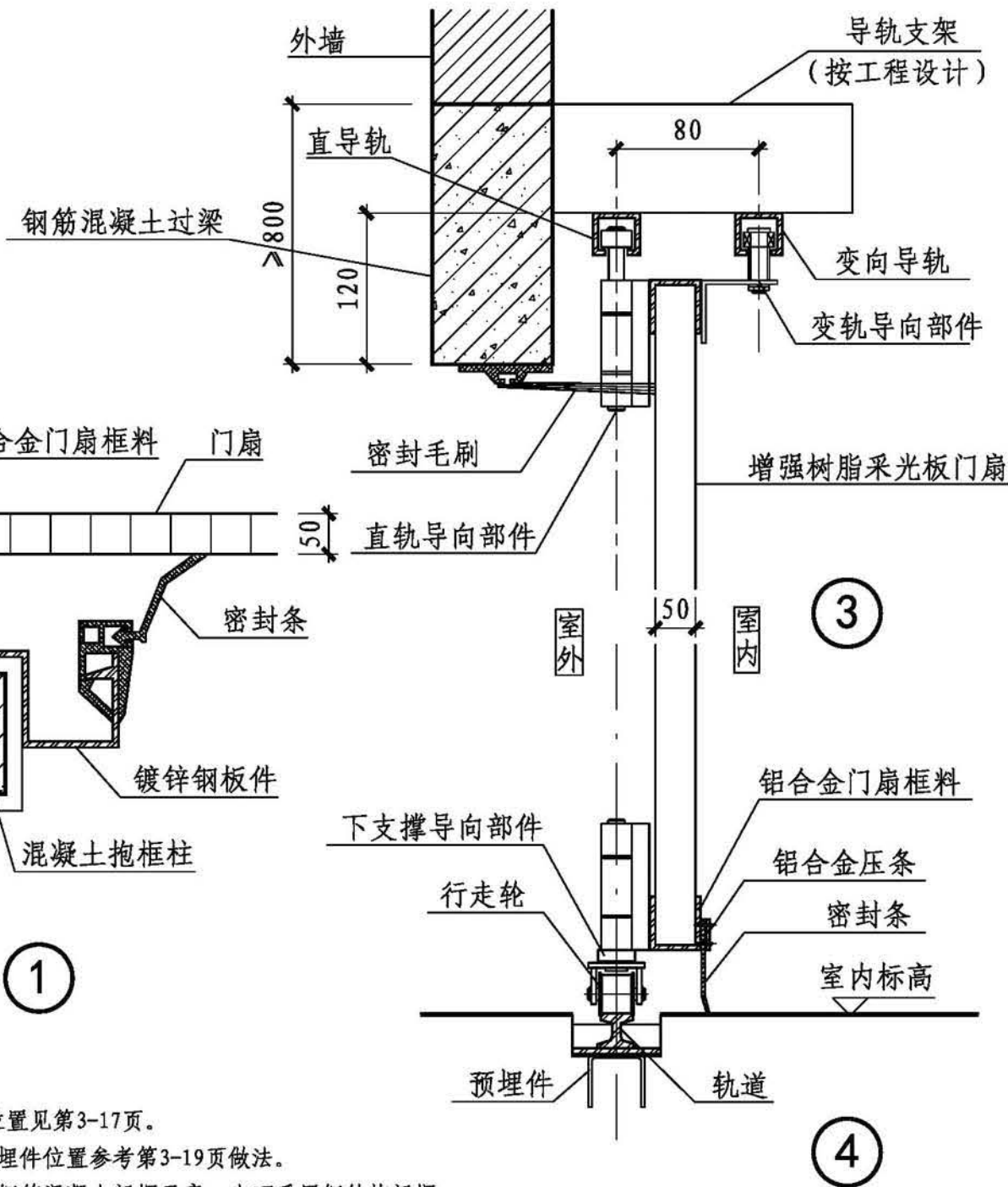
增强树脂板侧叠门剖面图、详图
