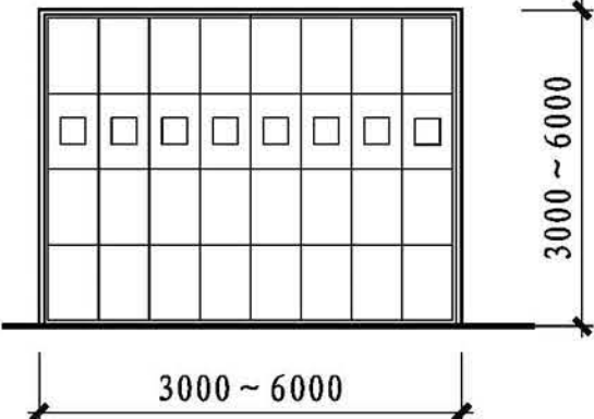
滑升门
